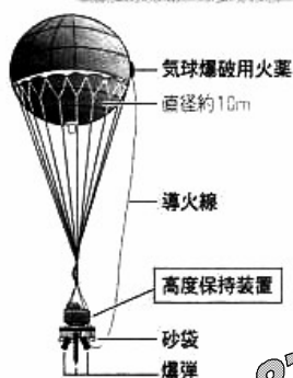
風船爆弾の完成図
